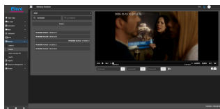
Memory Browser
